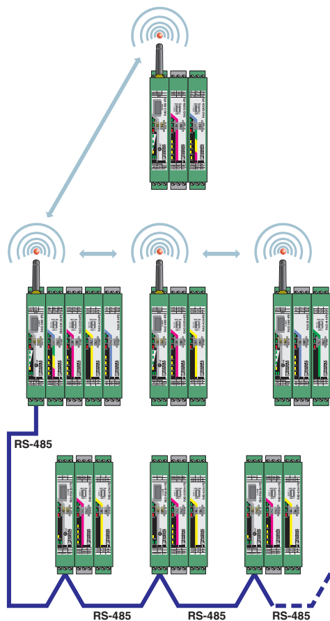
Funktionszeichnung
