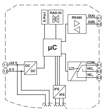
Blockschaltbild
