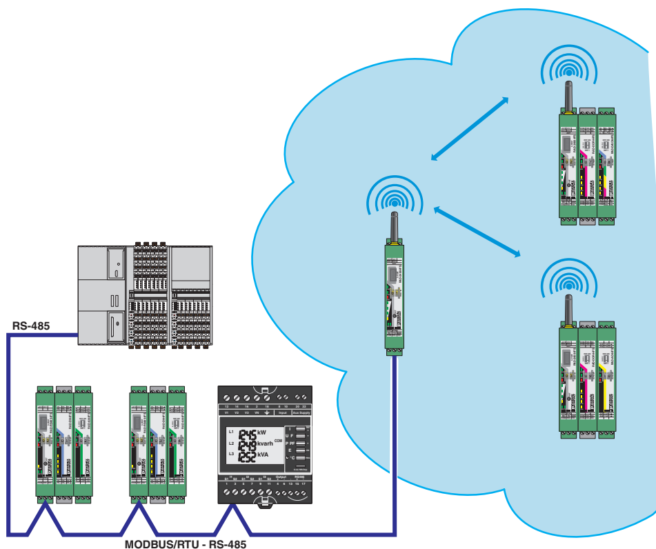
Radioline-Funksystem und RS-485-Stationen an einem Modbus-Master (I/O-zu-seriell)
