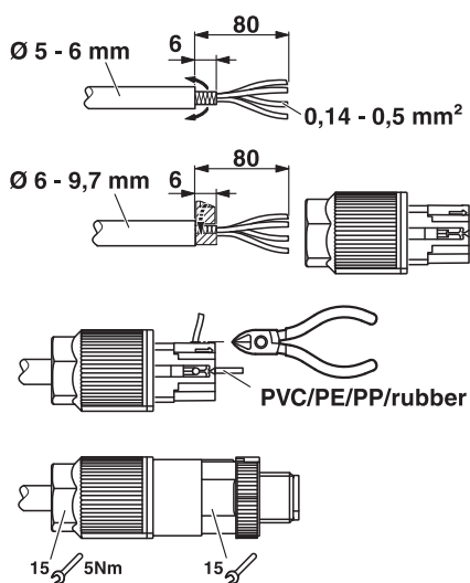
Funktionszeichnung
