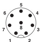
Polbild Stecker M12, 8-polig, A-kodiert, Ansicht Steckerseite
