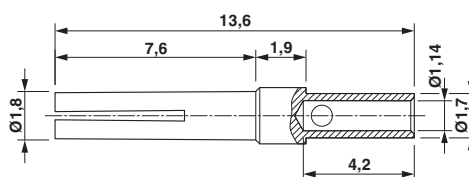
Maßzeichnung
