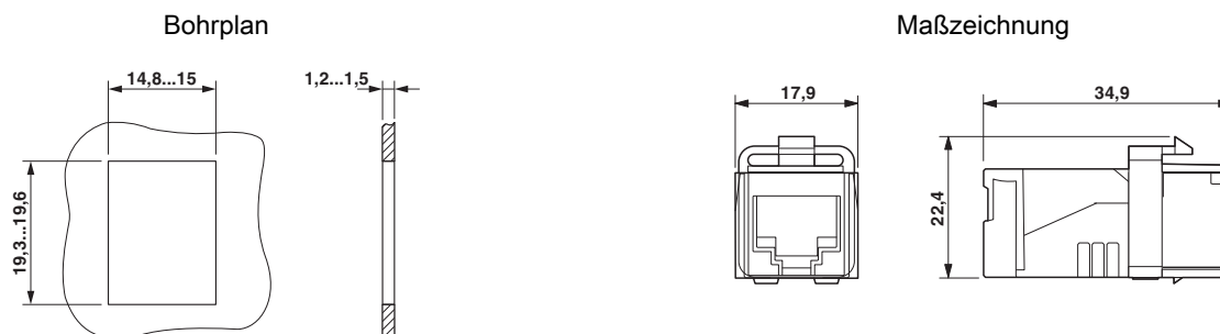
RJ45-Buchseneinsatz, Keystone
