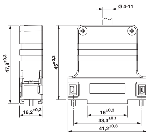
D-SUB-Tüllengehäuse
