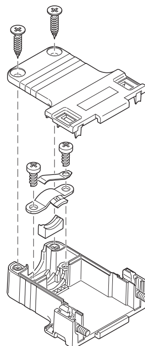
Schemazeichnung
