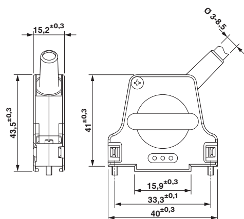
Maßzeichnung
