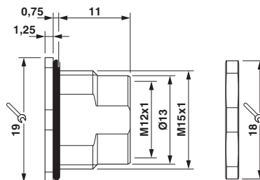
Maßzeichnung
