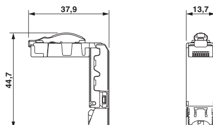
Maßzeichnung
