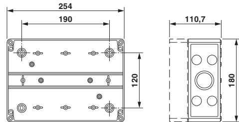
Maßzeichnung
