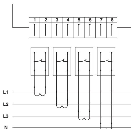
Schaltplan
