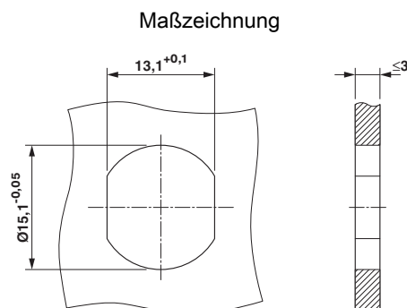
Gehäuseausschnitt mit Verdrehschutz
