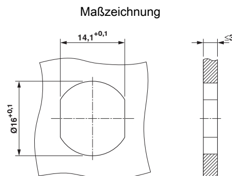
Gehäuseausschnitt mit Verdrehschutz. Gehäuseverschraubung vormontiert auf Isolierkörper mit anschließender Montage in der Frontplatte.
