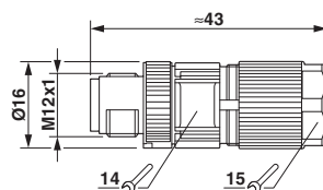
Maßzeichnung
