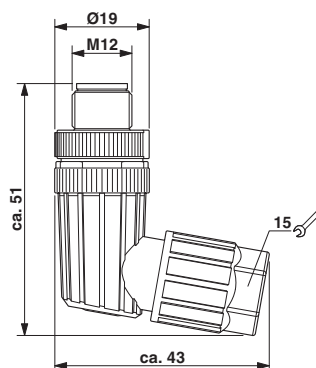
Maßzeichnung
