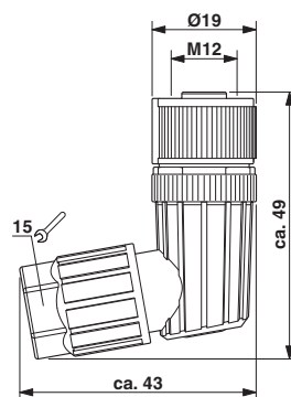
Maßzeichnung
