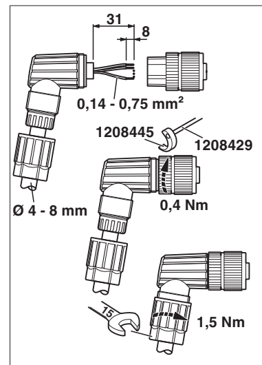
Funktionszeichnung
