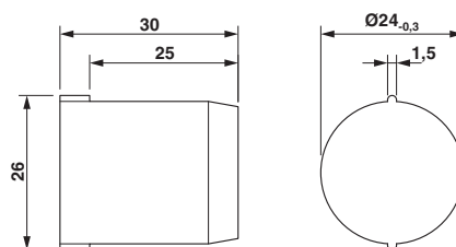
Maßzeichnung
