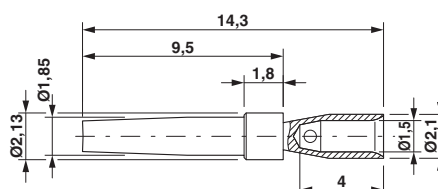
Maßzeichnung
