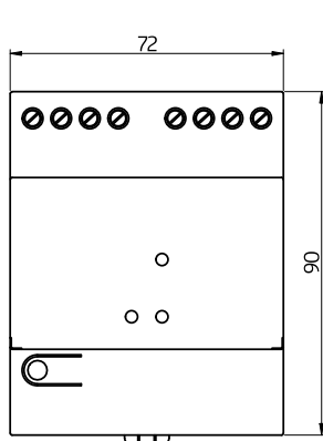
Bemaßung 93189
