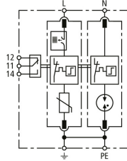
Principalschaltbild DG M TN ACI 275 FM
