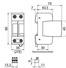
Maßbild DG M TN ACI 275 FM
