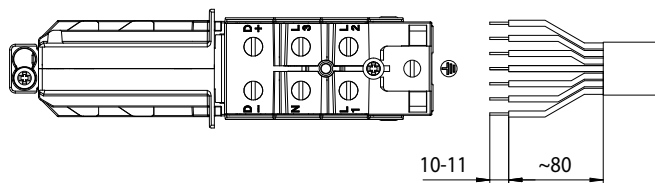
Abb. 3 Länge der Leiter Pic. 3 Length of the wires
