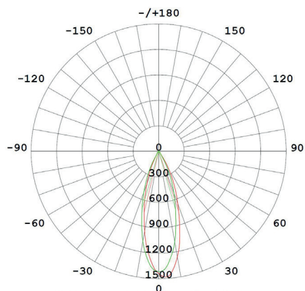
Lichtstärkeverteilung
