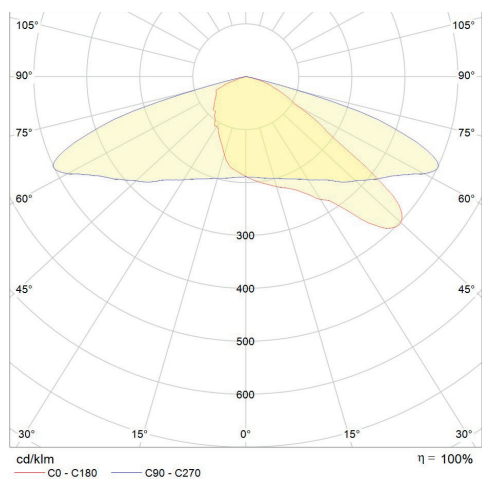
Polardiagramm
