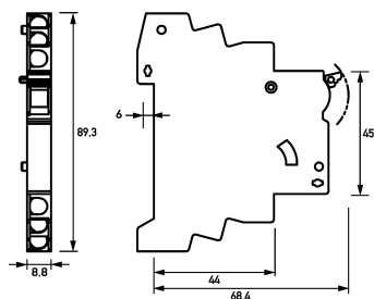
Maßzeichnung Hilfsschalter DHi 8 H10UM
