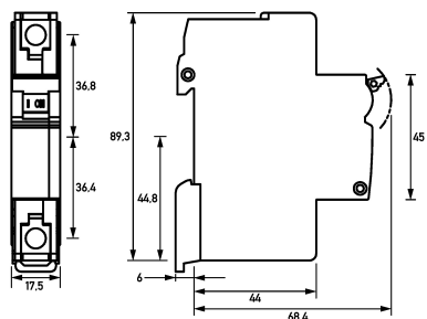
Maßzeichnung Manual Motor Controllers DLS 8 1C2UM
