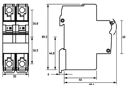
Maßzeichnung Manual Motor Controllers DLS 8 2E5UM
