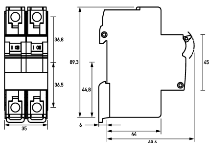
Maßzeichnung Manual Motor Controllers DLS 8 2Z05UM
