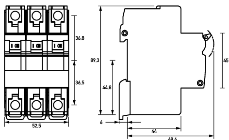
Maßzeichnung Manual Motor Controllers DLS 8 3D12UM
