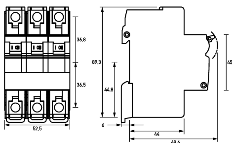
Maßzeichnung Manual Motor Controllers DLS 8 3G5UM
