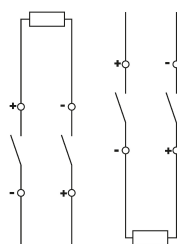
Schaltungsbeispiel Leitungsschutzschalter DLS 6hdc B63-2
