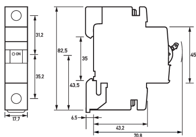
Maßzeichnung Leitungsschutzschalter DLS 6hdc C6-1
