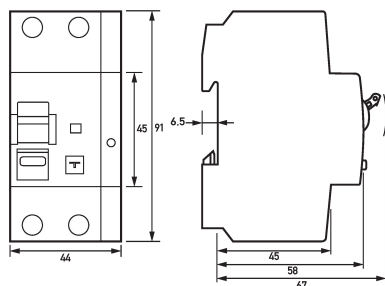
Maßzeichnung FI-/LS-Kombinationen DRCBO 4 B20/0,03/1N-B NK
