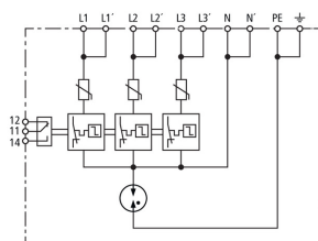
Prinzipschaltbild DCOR 3P TT 275 FM
