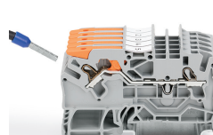
Direktes Stecken (Push-in) – feindrätige Leiter mit Aderendhülse
