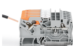
Direktes Stecken (Push-in) – eindrätige Leiter
