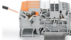
Direktes Stecken (Push-in) – eindrängige Leiter
