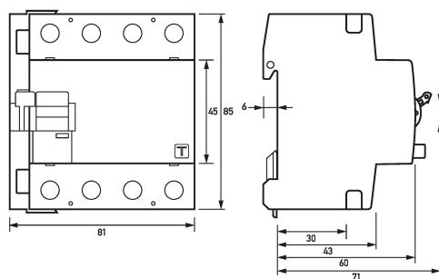
Mazeichnung Fehlerstromschutzschalter DFS 4 080-4/0,03-B SK NA
