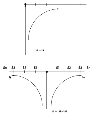
Diagramme Verdrahtungsmaterial BG4.2.10
