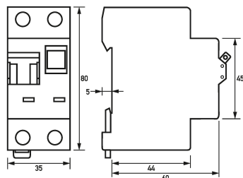
Maßzeichnung FI-/LS-Kombinationen DRCBO 3 Bo6/0,30/1N-A
