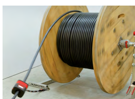
RM35 mit RUNPOLIFER L1600 und 3 x 35 mm 2 Kabel
