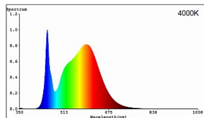
LED-NEO-Tubes 4000K, Ersatz für Leuchtstofflampen
