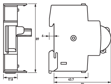
Maßzeichnung automatisch wiedereinschaltende Einrichtungen DFA 3 012DC-0
