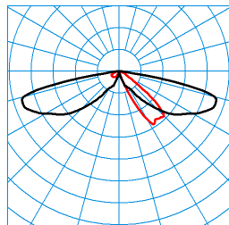
8841 AB2L/700-730 2G2 ETDD (CLOENDWERT) TX369233 DIN 5040: A20 UTE: 1,00 J CEN Flux Code: 20 59 92 100 100 0 0 0 0 ■ C0 - C180 ■ C90 - C270
