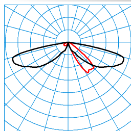
8841 AB2L/700-730 2G2 ETDD (CLOANFANGSWERT) TX369326 DIN 5040: A20 UTE: 1,00 J CEN Flux Code: 20 59 92 100 100 0 0 0 0 ■ C0 - C180 ■ C90 - C270
