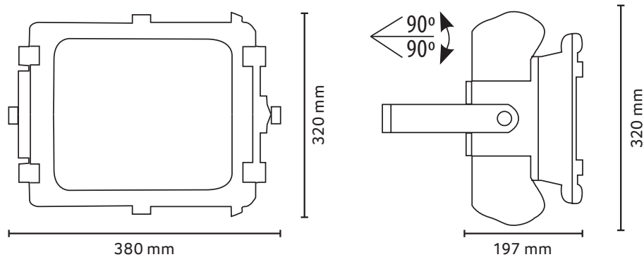
Abmessungen Leuchte
