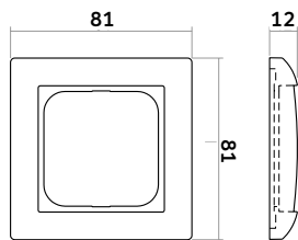
Abdeckrahmen 1-fach
