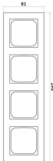
Abdeckrahmen 4-fach
