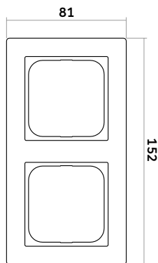
Abdeckrahmen 2-fach
