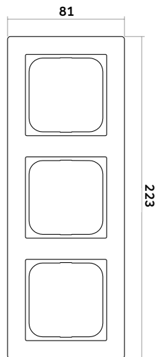
Abdeckrahmen 3-fach
