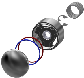
Druckkappe
