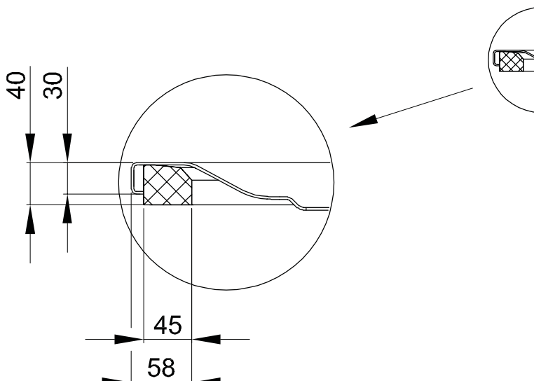
Darstellung mit vormontiertem Minimum-Wannenträger (T1).
