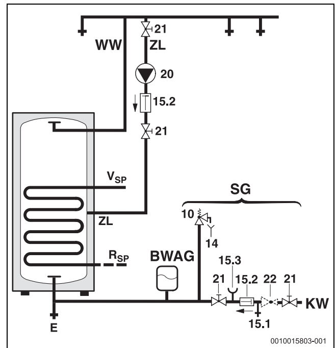
Fig. 4 Diagrama de conexión de agua potable
