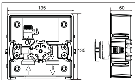
Abb. 3: Maße in mm
