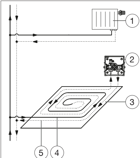
Abb. 10: Anschluss
