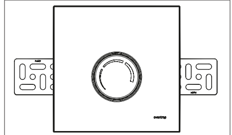
Abb. 11: „Unibox RTL vario“ mit Winkeln
