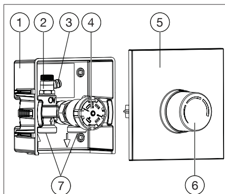
Abb. 2: Aufbau „Unibox RTL vario“
