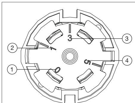
Abb. 6: Einstellmöglichkeiten Fühlereinheit
