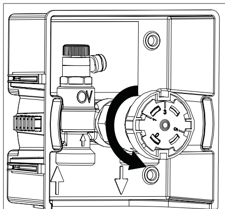
Abb. 17: Thermostat „RTL vario“ abschrauben
