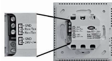
Anschlussklemmen KaController
