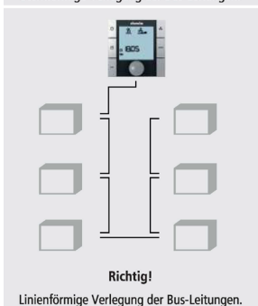
Verlegung der Bus-Leitungen
