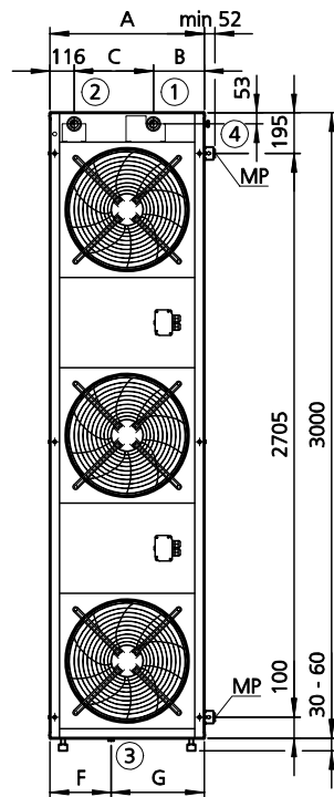
Seitenansicht Typ 23020**
