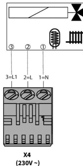
Abb. 21: Anschluss 3-Wege-Umschaltventil
