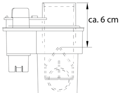
Abb. 100: Korrekte Position von Sicherungsklammer und Kunststoffkugel
