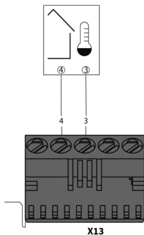
Abb. 19: Anschluss Außentemperaturfühler
