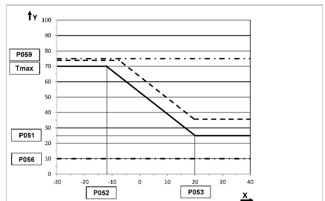
Abb. 90: Heizkennlinie mit Parallelverschiebung (T RaumSoll = 24°C, P054 = 3) und Begrenzung durch Parameter P059
