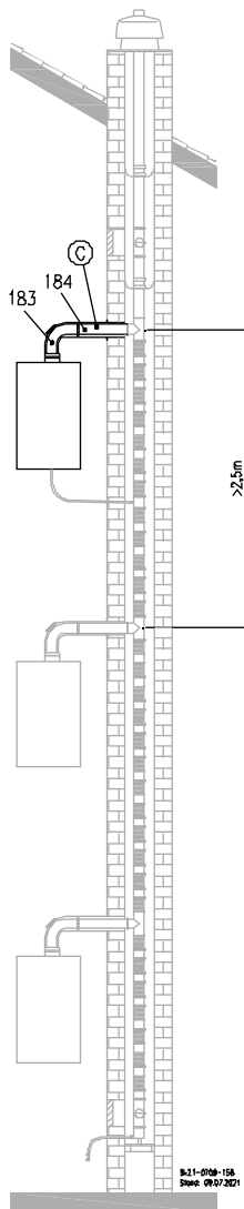
Abb. 40: C (10)3x Mehrfachbelegung im Schacht
