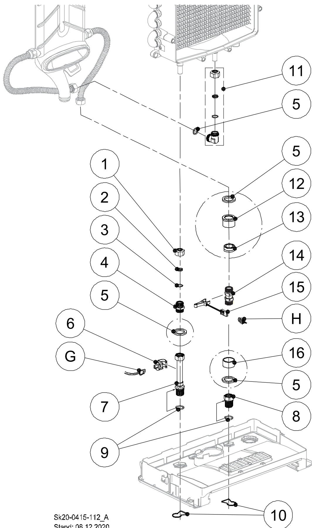
Abb. 111: Hydraulik Trinkwasser
