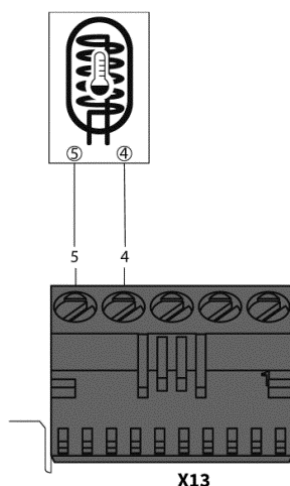
Abb. 20: Anschluss Trinkwarmwasserspeicher-Temperaturfühler
