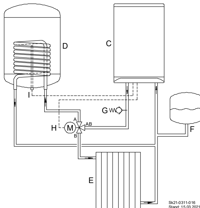
Abb. 22: Trinkwarmwasserbereitung mit externem Speicher über 3-Wege-Umschaltventil
