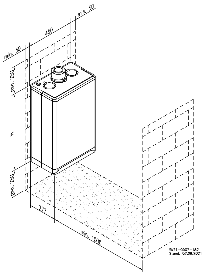
Abb. 3: Montageabstände
