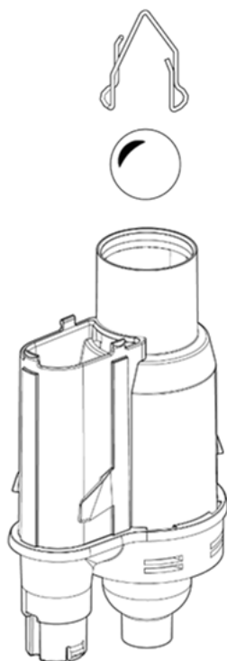
Abb. 99: Sicherungsklammer und Kunststoffkugel des Siphons
