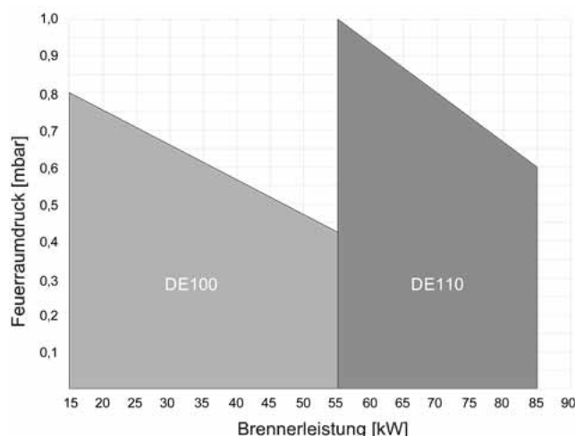
Abb. 20: Leistungsdiagramm
