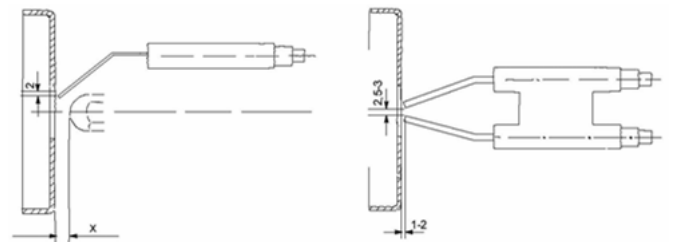
Abb. 12: Zündelektrodeneinstellung
