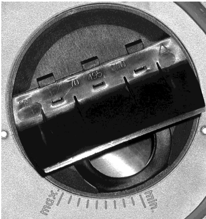
Abb. 10: Lufteinlaufdüse
