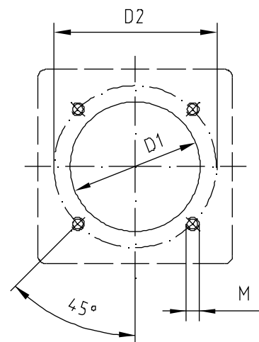
Abb. 2: Kesselanschluss
