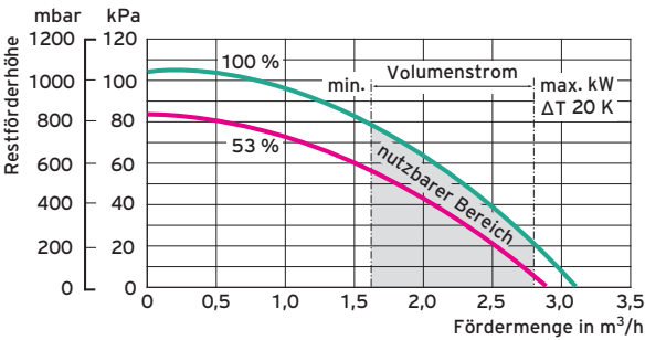
Pumpendiagramm VC 656
